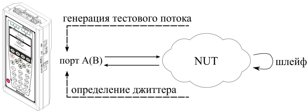
Рисунок 10.30. Измерение джиттера. Схема 1
