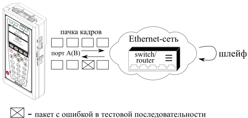
Рисунок 10.28. Тестирование на канальном/сетевом уровне (вариант 2)
