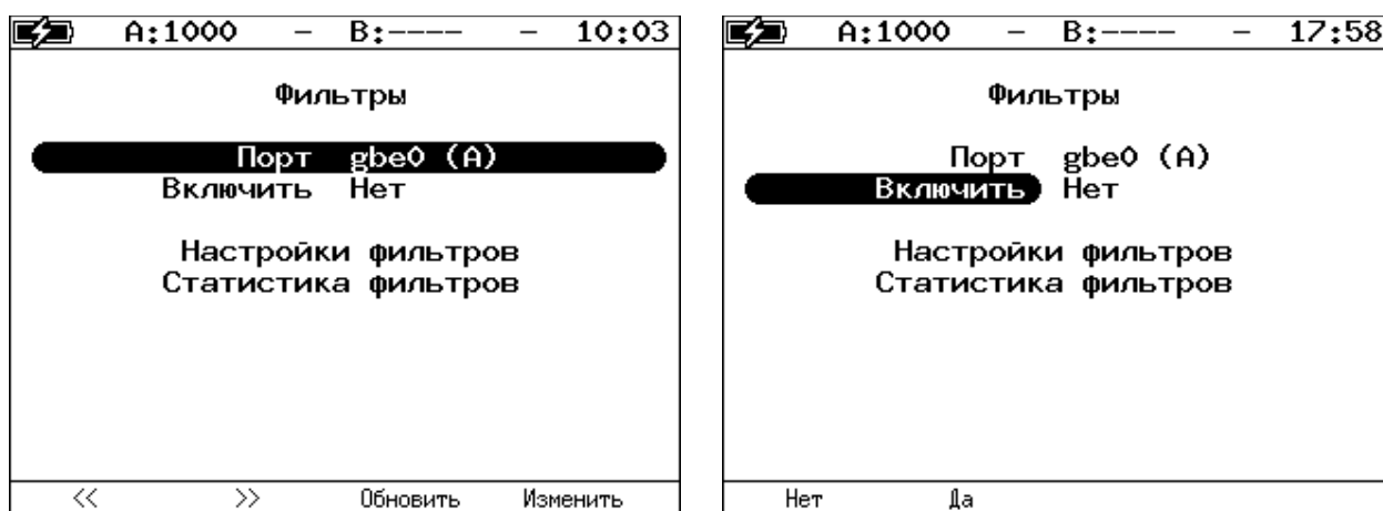
Рисунок 16.33. Меню «Фильтры»
