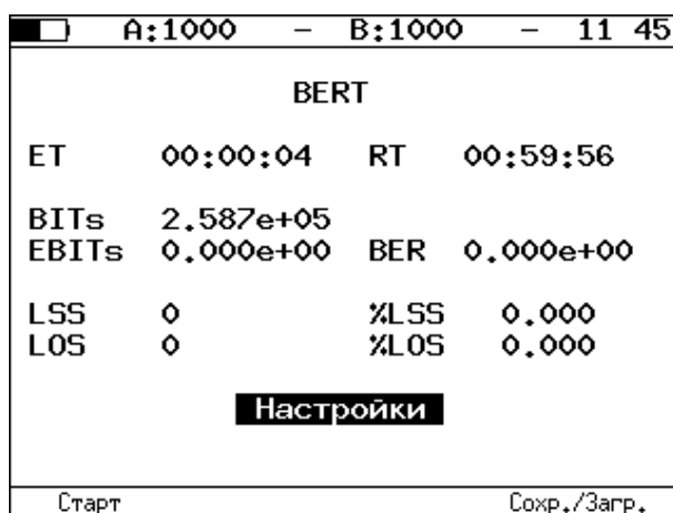
Рисунок 17.33. Меню «BERT»
