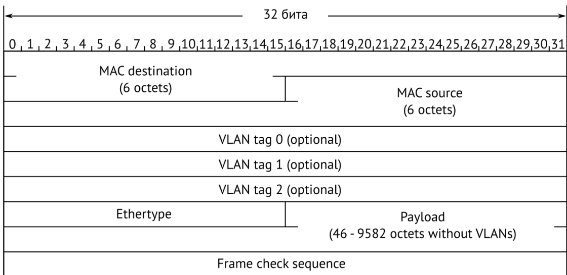
Рисунок 28.2. Структура кадра 2-го уровня
