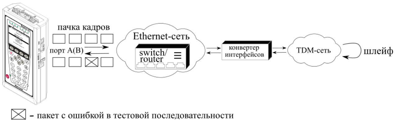
Рисунок 10.27. Тестирование на канальном/сетевом уровне (вариант 1)
