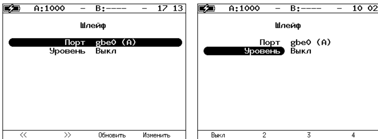
Рисунок 16.31. Меню «Шлейф»
